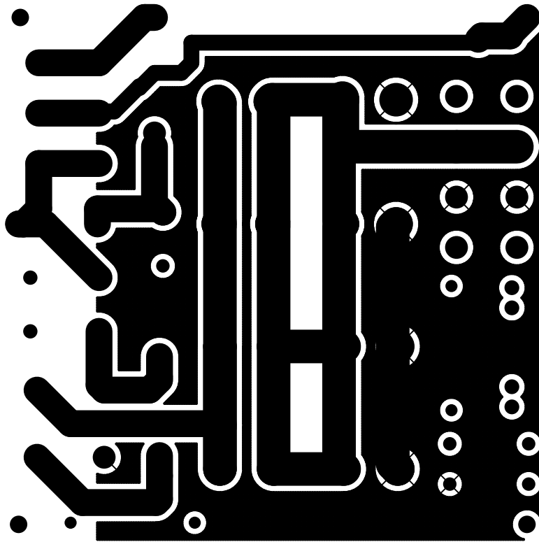
TOP LAYER
