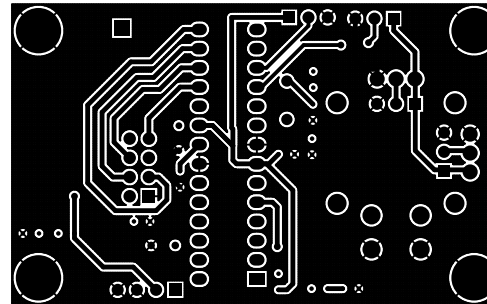
BOTTOM LAYER
