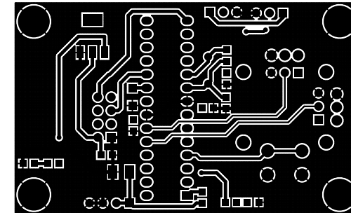
TOP LAYER
